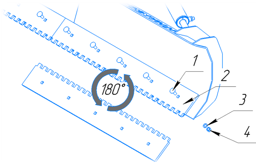
Рис 13. Замена ножей отвала
