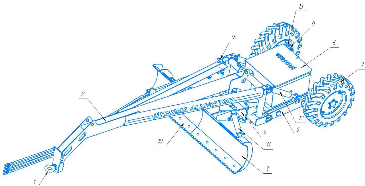
Рис.1. Общее устройство
