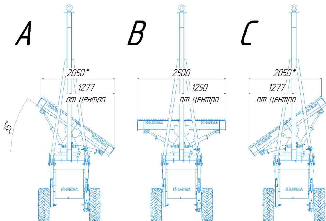
Рис.10 Ширина захвата при повороте отвала на 35^\circ
