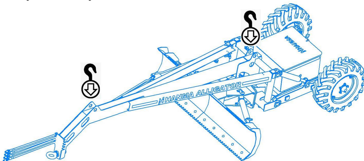
Рис.9 Схема строповки прицепного грейдера
