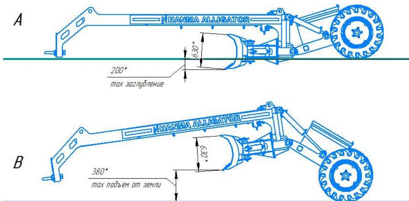
Рис.11 Глубина опускания и высота подъема
