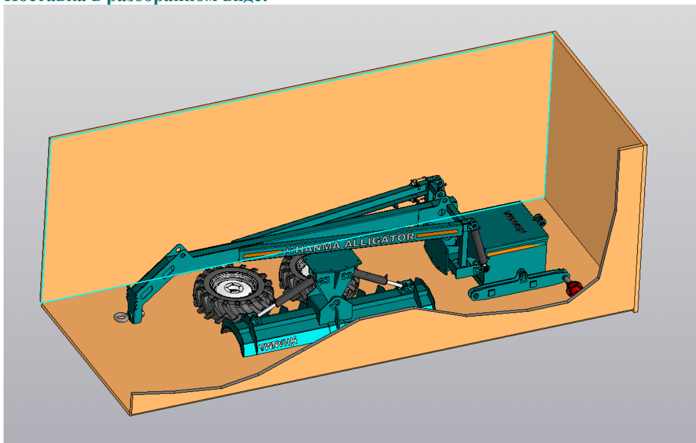
Рис.5 Рекомендуемый вариант транспортировки прицепного грейдера в разобранном виде
