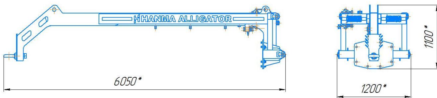
Рис.6 Габариты рамы в сборе
