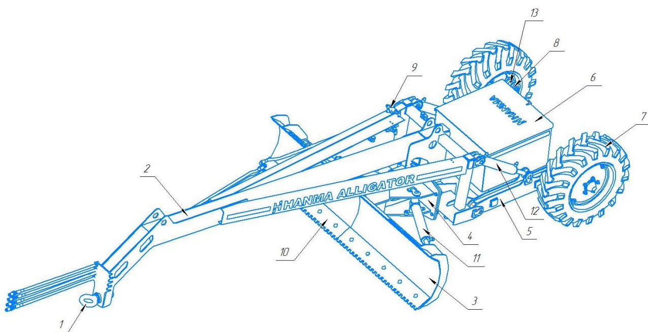
Рис.1 Общее устройство
