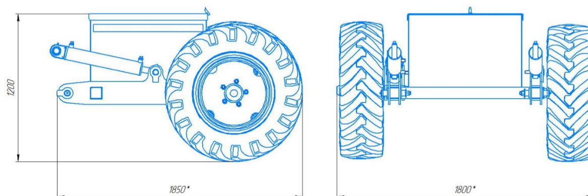
Рис.7 Габариты тележки в сборе
