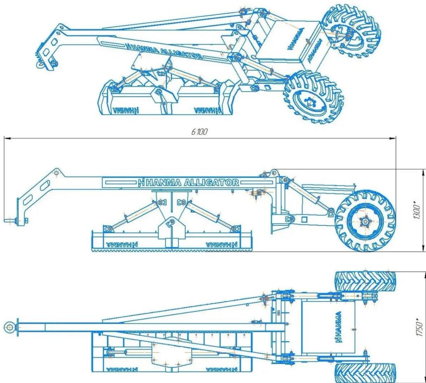
Рис.4 Габариты в собранном виде
