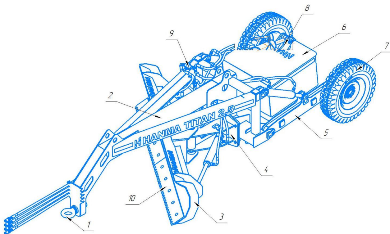
Рис.1 Общее устройство
