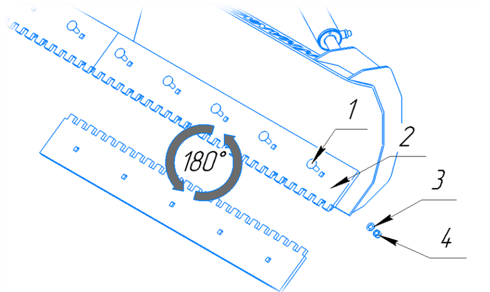
Рис.13 Замена ножей отвала
